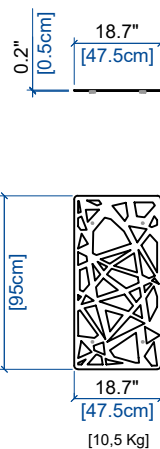
BTP PLATEFORME TABLETTE COFFEE TABLE PLATFORM PLATAFORMA MESA PEQUEÑA
