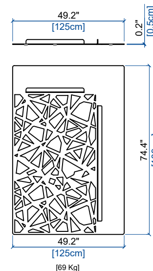
BHD PLATEFORME CHAISE LONGUE DROITE LOUNGE RIGHT SEAT PLATFORM PLATAFORMA CHAISE LONGUE DER.
