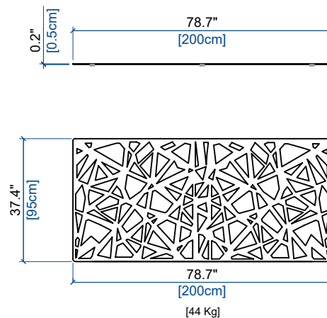
BTG TABLE BASSE RECTANGULAIRE RECTANGULAR TABLE MESA RECTANGULAR
