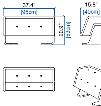
DOSSIER DROIT STRAIGHT BACK CUSHION COJIN DE RESPALDO RECTO
