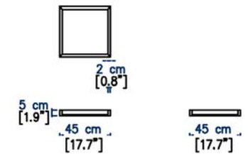
CA38 PLATEAU POUR TABLE BASSE TRAY FOR TABLE BANDEJA PARA MESA
