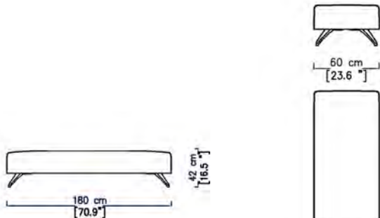
CA33 GRAND POUF RECTANGULAIRE MONOBLOC RECTANGULAR FOOTSTOOL MONOBLOC PUF RECTANGULAIRE MONOBLOC
