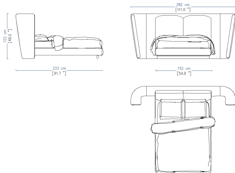
LIT 140x190 - Tête de lit en 2 parties BED 140x190 - Headboard in 2 parts CAMA 140x190 - Cabecero de cama 2 partes
