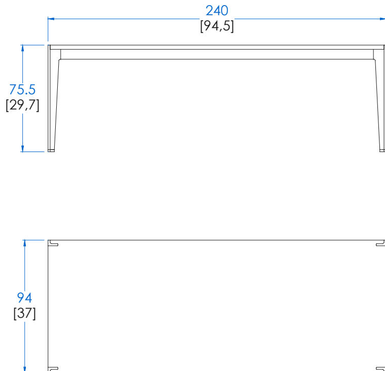
P.AS.MS041FCN - Table de Repas Fixe – L 240 H 75,5 P 94 cm
