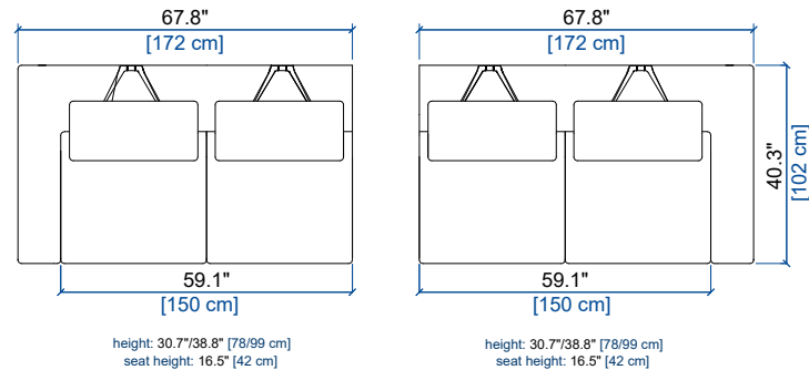
27 BATARD 2PL. ACC.GAUCHE 2-SEAT 1-ARM UNIT LEFT ARMREST BATARD 2 PL. APOY.IZQUIERDO
