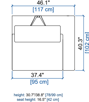
28 BATARD 1PL. ACC.DROIT 1-SEAT 1-ARM UNIT RIGHT ARMREST BATARD 1 PL. APOY.DERECHO
