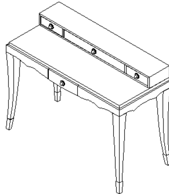
P.MC.MD04 – Écritoire - L 115 H 86 P 52 cm
