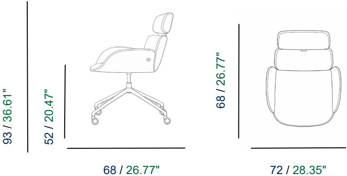
FAUTEUIL VISITEUR AVEC ROULETTES VISITOR ARMCHAIR WITH LOW BACK WITH CASTERS SILLÓN DE VISITANTE CON RUEDAS
