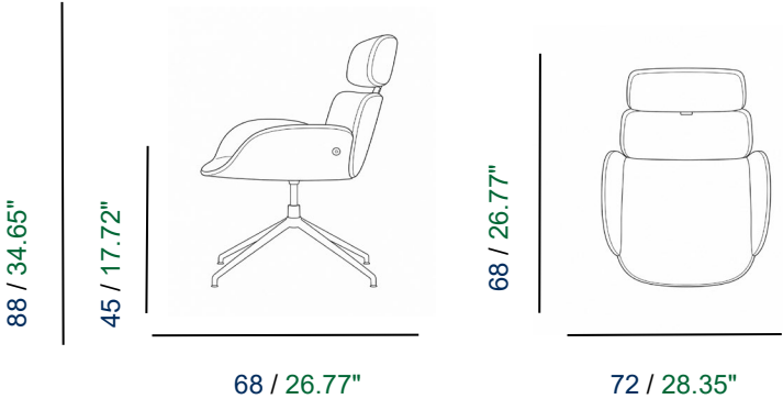
FAUTEUIL VISITEUR SANS ROULETTES VISITOR ARMCHAIR WITHOUT CASTERS SILLÓN DE VISITANTE SIN RUEDAS
