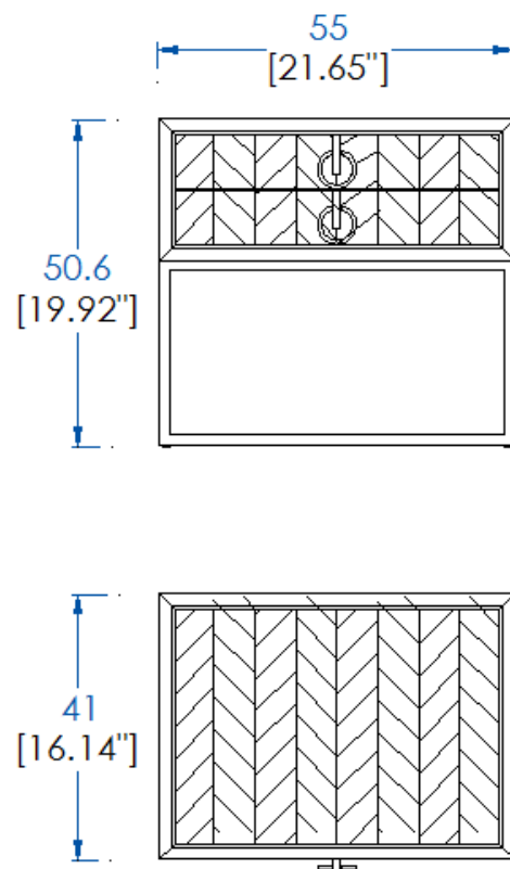
P.MT.CH02HI – Chevet 2 tiroirs – piétement inox – L 55 H 50.6 P 41 cm
