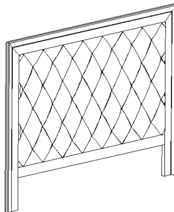
P.MT.CB08 – Tête de lit l. 193 - king size – capitonnée cuir - L 226.4 H 170 P 6 cm
