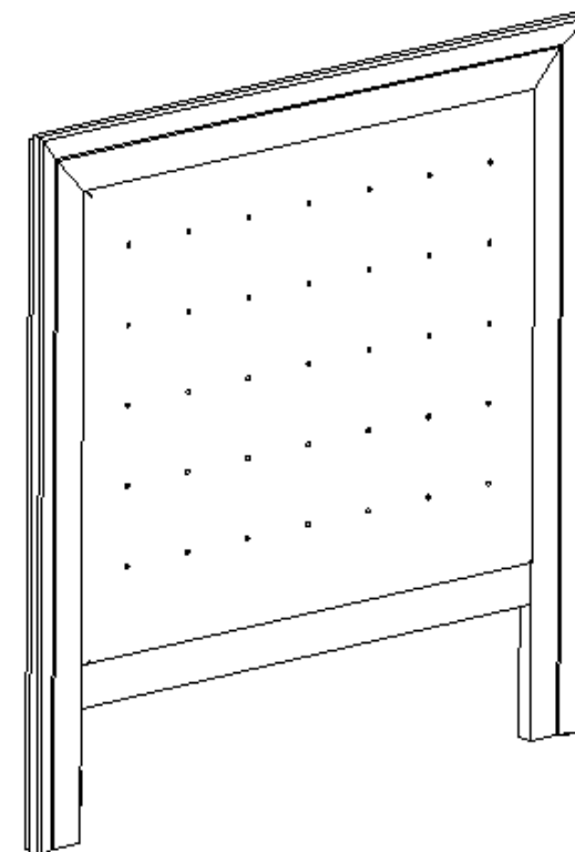
P.MT.CB02 – Tête de lit l.140 – capitonné vinyl - L 173.4 H 170 P 6 cm
