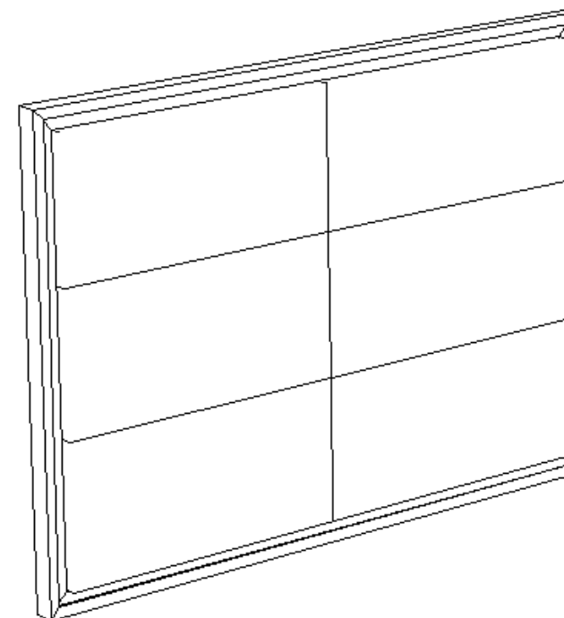
P.MT.CBE02 - Tête de lit l.140 - garnie vinyl - L 180 H 140 P 8 cm
