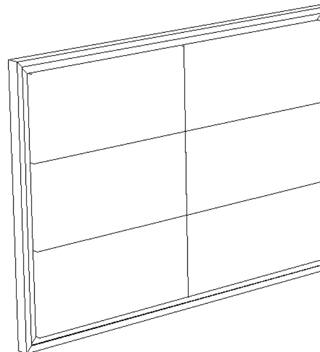
P.MT.CBE03 - Tête de lit l180 - garnie vinyl - L 220 H 140 P 8 cm
