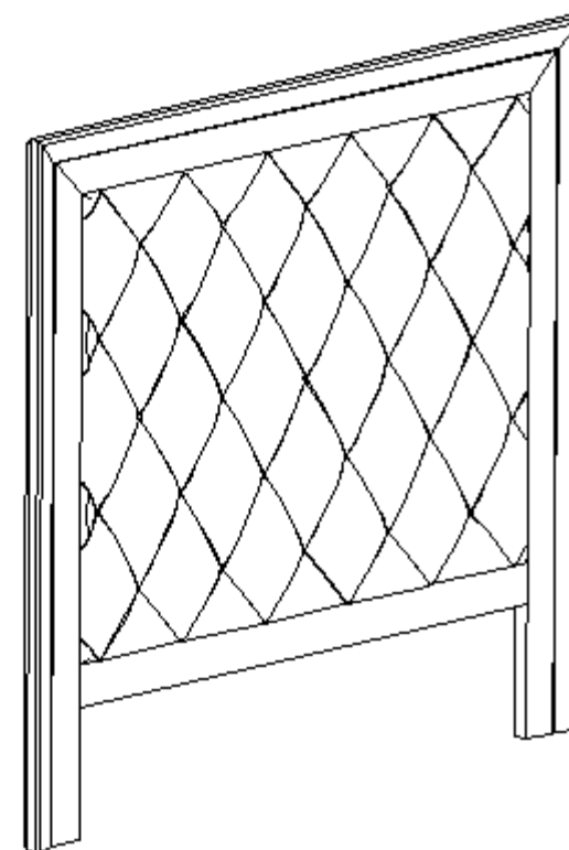
P.MT.CB02 – Tête de lit l.140 – capitonnée cuir - L 173.4 H 170 P 6 cm
