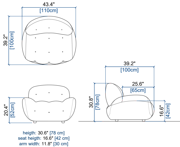
FAUTEUIL ARMCHAIR SILLON
