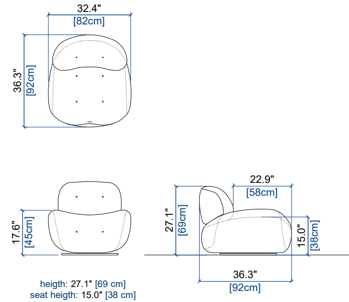
FAUTEUIL PIVOTANT SWIVEL ARMCHAIR SILLON GIRATORIO
