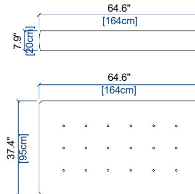
ASSISE CHAISE LONGUE CHAISE LONGUE SEAT CUSHION ASIENTO CHAISE LONGUE
