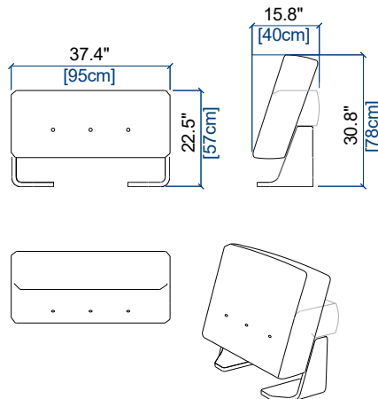
DOSSIER DROIT AVEC MECANISME STRAIGHT BACK CUSHION WITH MECHANISM COJÍN DE RESPALDO CON MECANISMO
