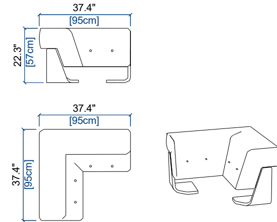
DOSSIER D'ANGLE BACK CORNER CUSHION COJÍN DE RESPALDO DE ANGULO
