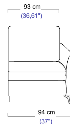
101 BATARD 1 PLACE ACC. DROIT 1-SEAT 1-ARM UNIT RIGHT BATARD 1 PLAZA DERECHO
