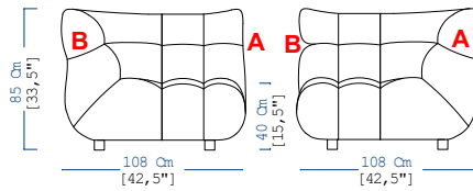
BATARD 1 PLACE GAUCHE 1-SEAT 1-ARM UNIT LEFT BATARD 1 PLAZA IZQUIERDO
