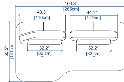
277 GRANDE BANQUETTE DOUBLE PROF.GAUCHE LARGE ARMLESS UNIT DOUBLE DEPHT LEFT GRAN BANQUETA DOBLE PROF.IZQDA
