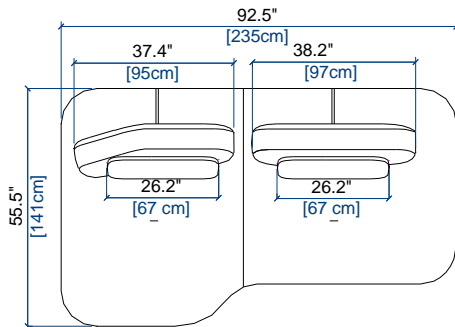
279 MOYEN BANQUETTE DOUBLE PROF.GAUCHE MEDIUM ARMLESS UNIT DOUBLE DEPHT LEFT MEDIA BANQUETA DOBLE PROF.IZQDA
