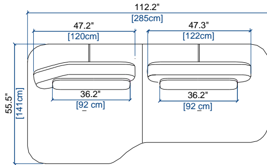
273 MAXI BANQUETTE DOUBLE PROF.GAUCHE MAXI ARMLESS UNIT DOUBLE DEPHT LEFT MAXI BANQUETA DOBLE PROF.IZQDA
