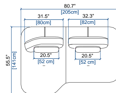
292 PETITE BANQUETTE DOUBLE PROF.GAUCHE SMALL ARMLESS UNIT DOUBLE DEPHT LEFT PEQUEÑA BANQUETA DOBLE PROF.IZQDA
