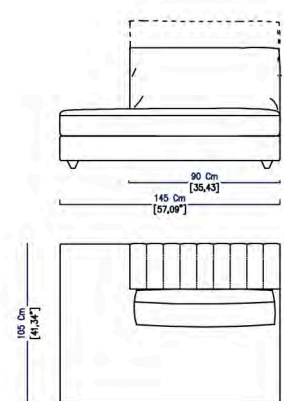
IM10 - PETIT TERMINAL GAUCHE DOSSIER RELEVABLE IM10 - SMALL END UNIT LEFT ADJUSTABLE BACK IM10 - PEQUENO TERMINAL IZQUIERDO RESPALDO ELEVABLE
