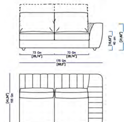
IM09 - BATARD 2 PLACES ACC. DROIT DOSSIERS RELEVABLES IM09 - 2-SEAT 1-ARM UNIT RIGHT ARMREST ADJUSTABLE BACKS IM09 - BATARD 2 PL. APY DERECHO RESPALDOS ELEVABLES
