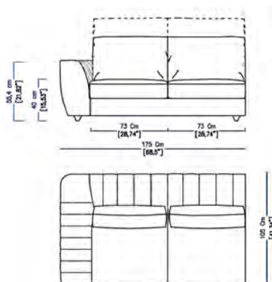
IM08 - BATARD 2 PLACES ACC. GAUCHE DOSSIERS RELEVABLES IM08 - 2-SEAT 1-ARM UNIT LEFT ARMREST ADJUSTABLE BACKS IM08 - BATARD 2 PL. APY IZQUIERDO RESPALDOS ELEVABLES
