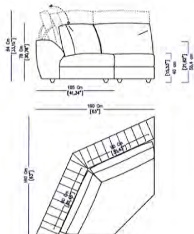
IM12 - ANGLE OUVERT DOSSIERS RELEVABLES IM12 - OPEN CORNER ADJUSTABLE BACKS IM12 - ANGULO ABIERTO RESPALDOS ELEVABLES
