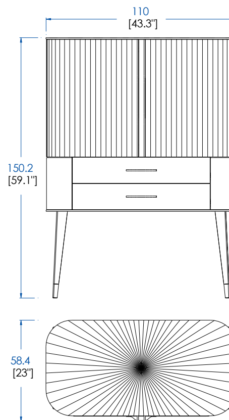
P.ER.AR02S – Meuble de rangement - plateau soleil – L 110 H 150.2 P 58.4 cm
