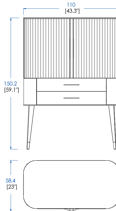
P.ER.AR02K – Meuble de rangement - plateau céramique carrare – L 110 H 150.2 P 58.4 cm
