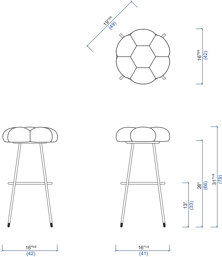
07 Tabouret de Bar haut High Bar Stool Taburete de bar alto
