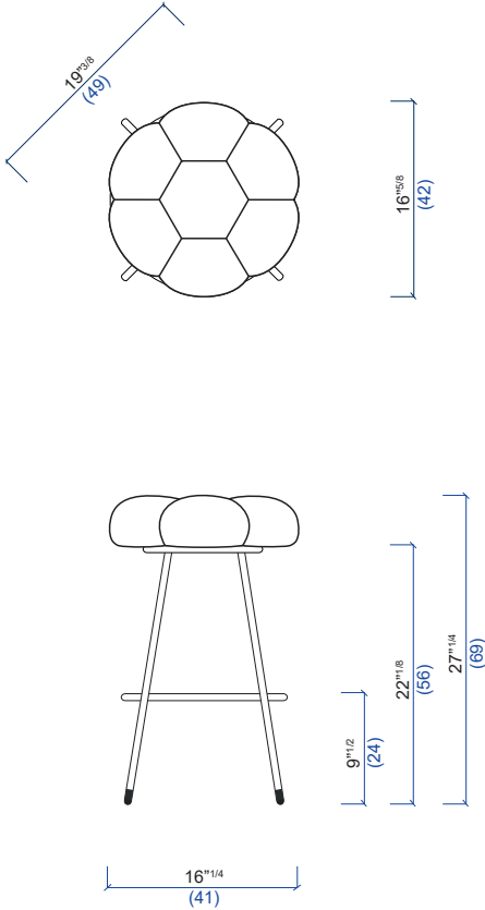
06 Tabouret de Bar bas Low Bar Stool Taburete de bar bajo
