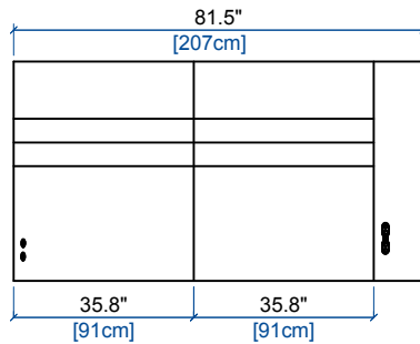
106 BATARD 3 PL. ACC. DROIT (EN 2 PARTIES) - FULL RELAX 3-SEAT 1-ARM UNIT RIGHT ARM. (IN 2 PARTS) - FULL RELAX BATARD 3 PL. APOY. DER. (EN 2 PARTES) - FULL RELAX
