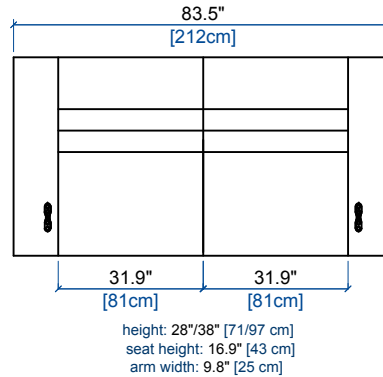
CANAPE 3 PLACES (EN 2 PARTIES) - FULL RELAX 3-SEAT SOFA (IN 2 PARTS) - FULL RELAX SOFA 3 PLAZAS (EN 2 PARTES) - FULL RELAX
