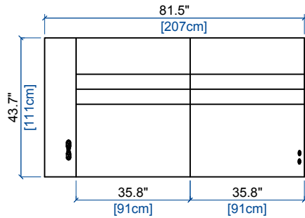
105 BATARD 3 PL. ACC. GAUCHE (EN 2 PARTIES) - FULL RELAX 3-SEAT 1-ARM UNIT LEFT ARM. (IN 2 PARTS) - FULL RELAX BATARD 3 PL. APOY. IZQ. (EN 2 PARTES) - FULL RELAX
